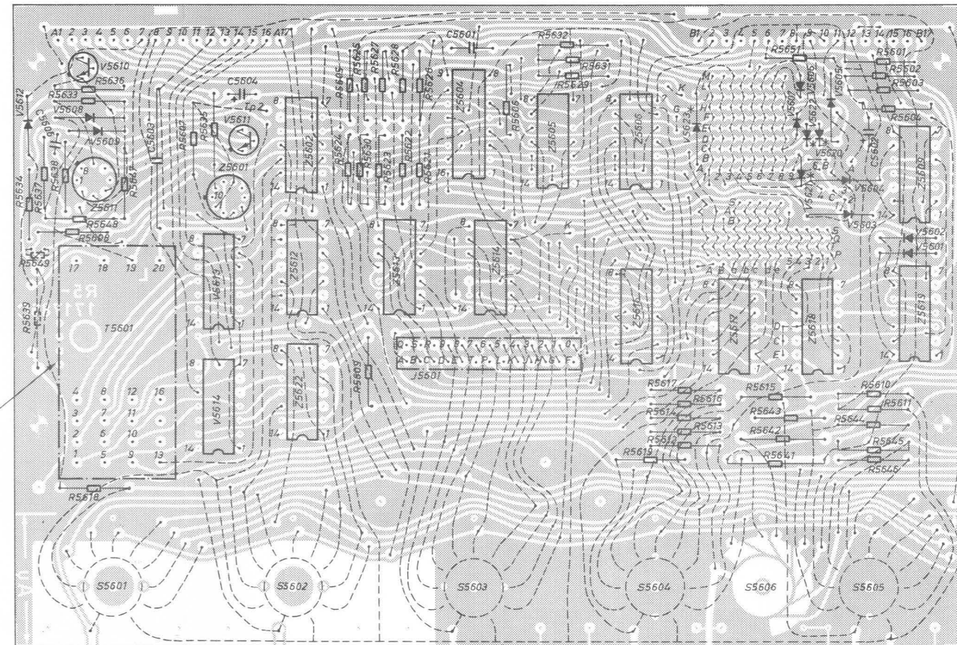
Komponentsida
