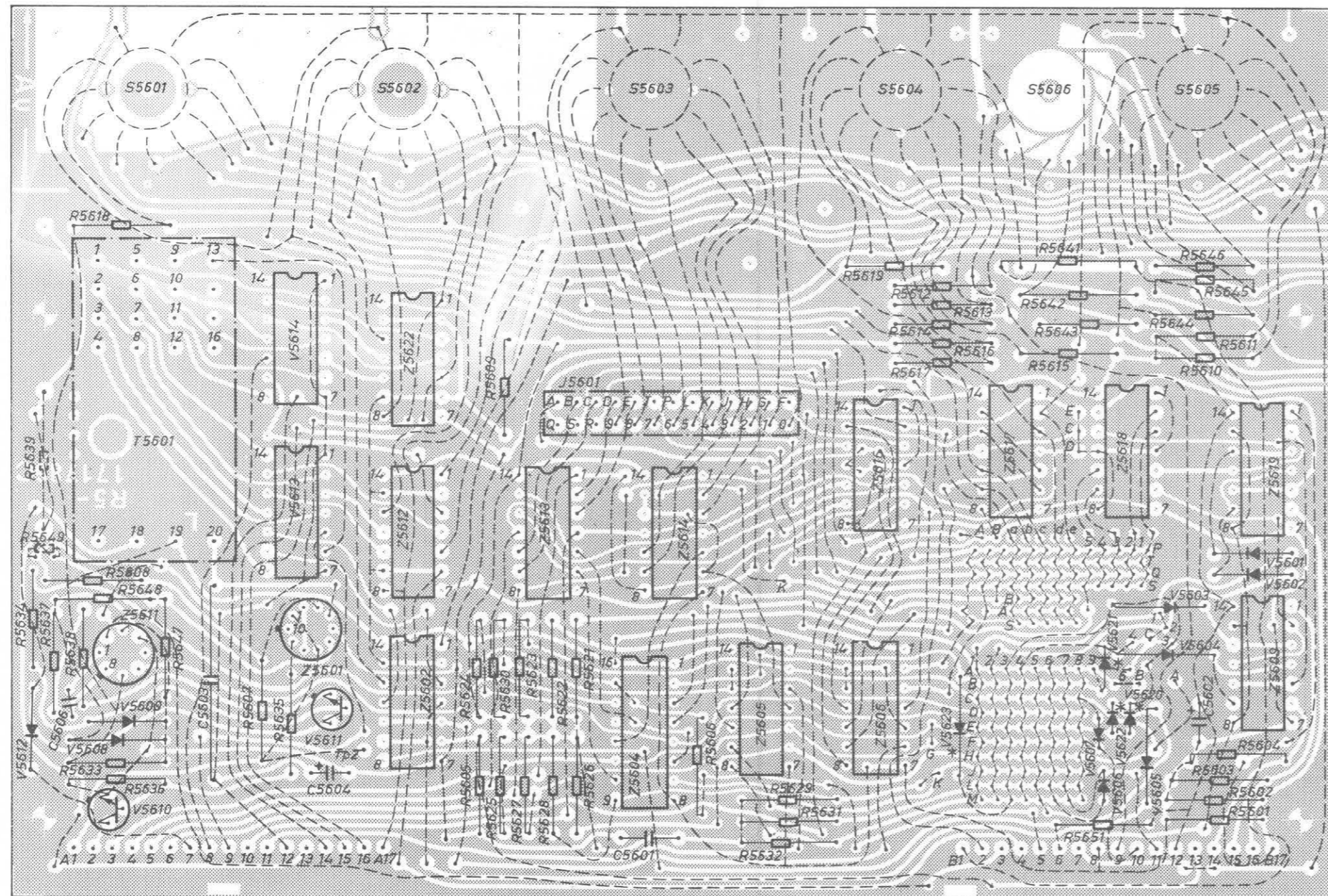
Lödsida
