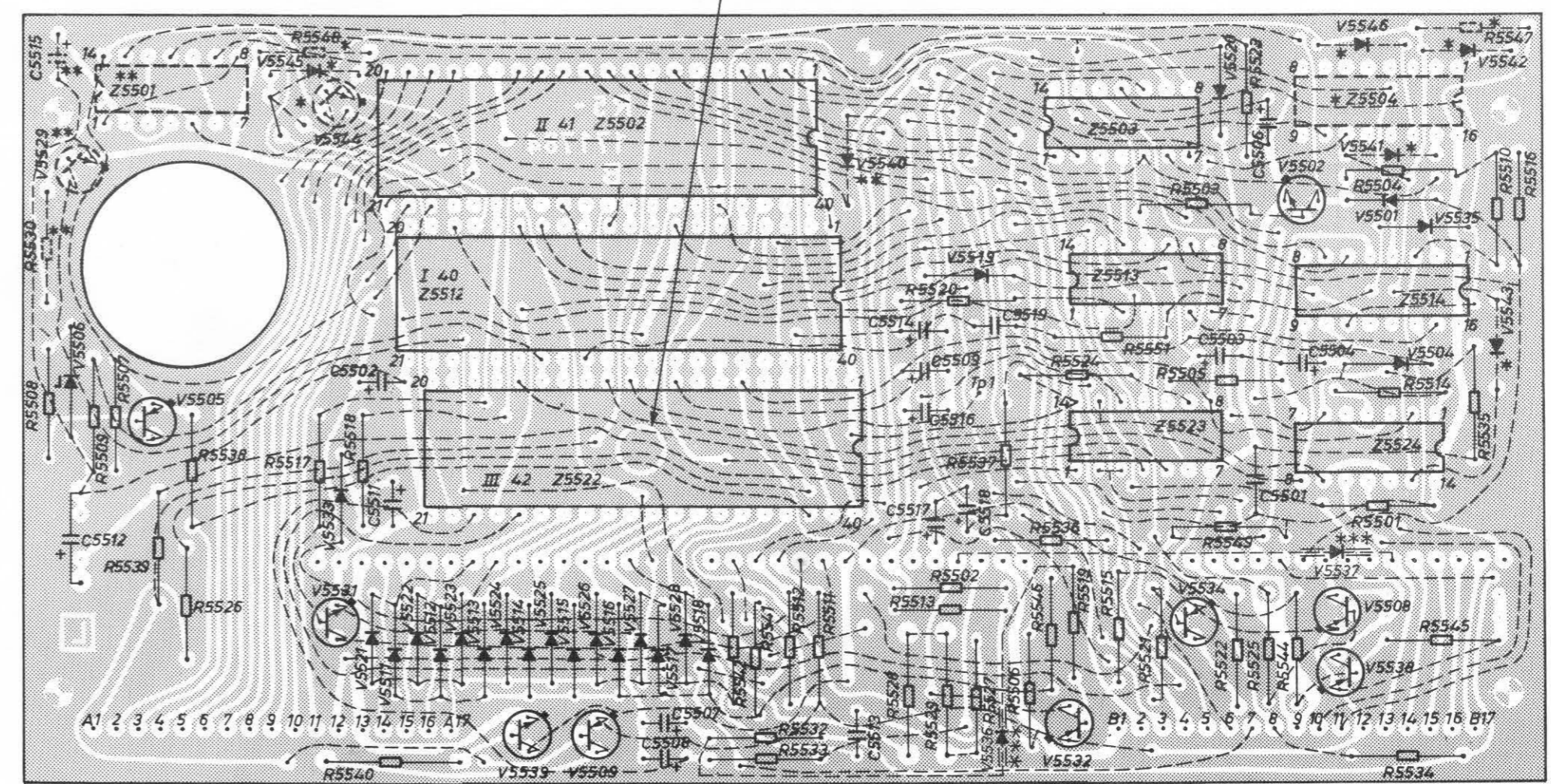
Komponentsida
