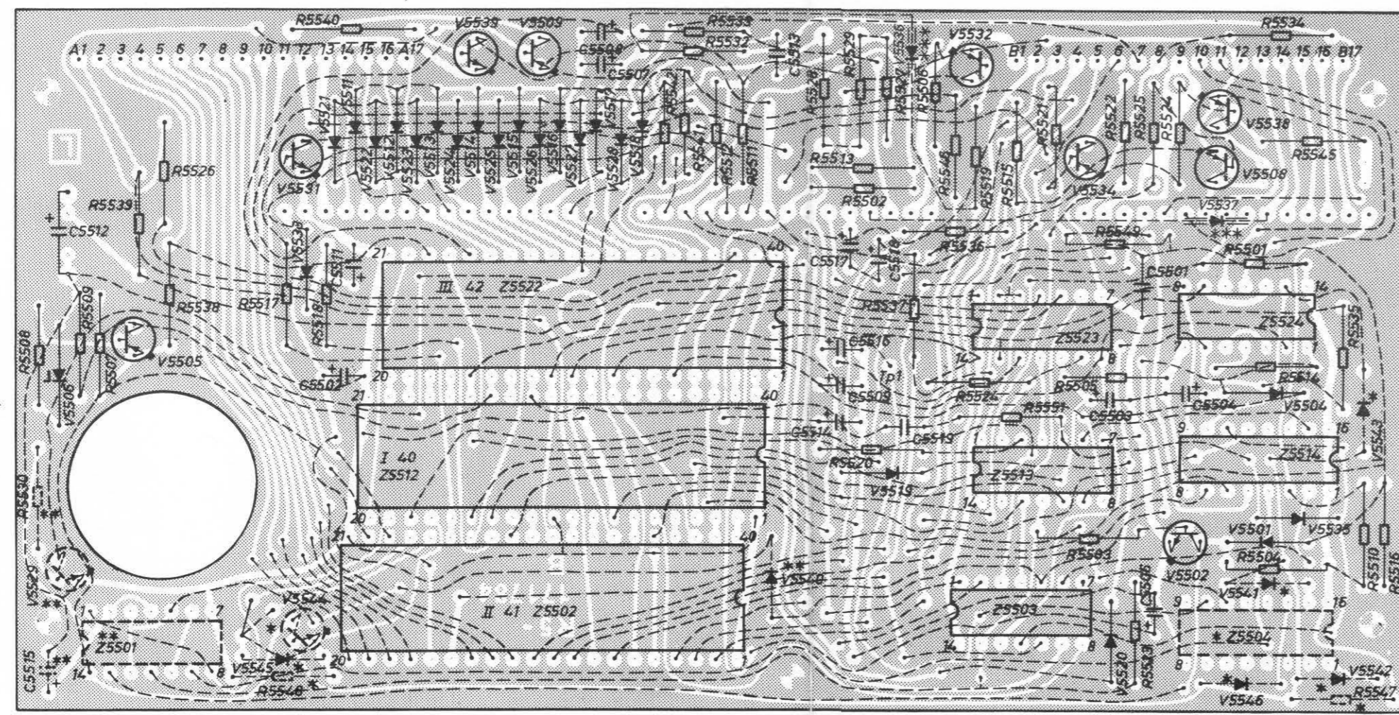
Lödsida
