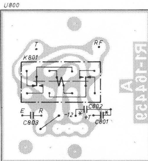
Komponentsida Component side Seite der Bauelemente Côté composants
