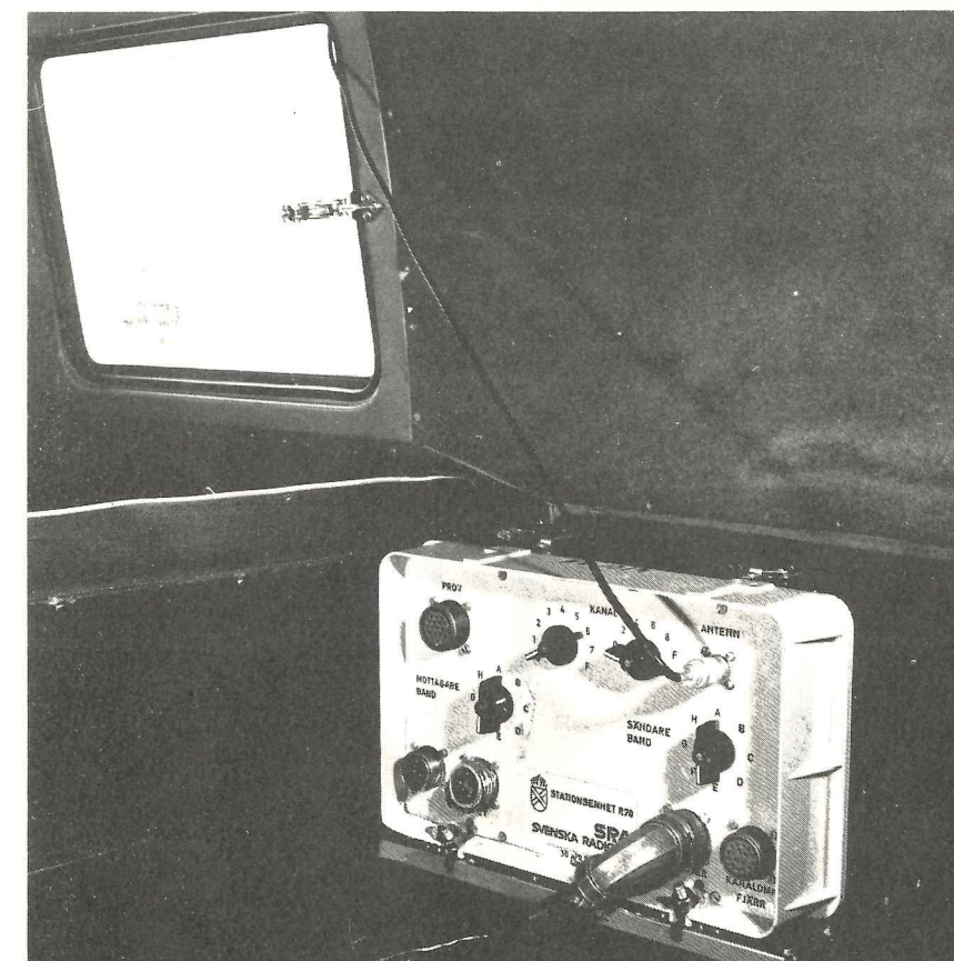
Fäst stationsenheten
